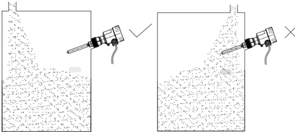
图 5 避开入料口的安装示意图
