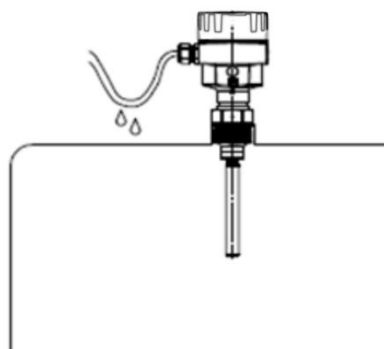
图 6 防潮安装
