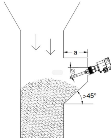
图 3 壁龛式安装示意图
