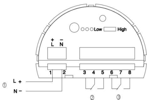
图 7 继电器输出方式
