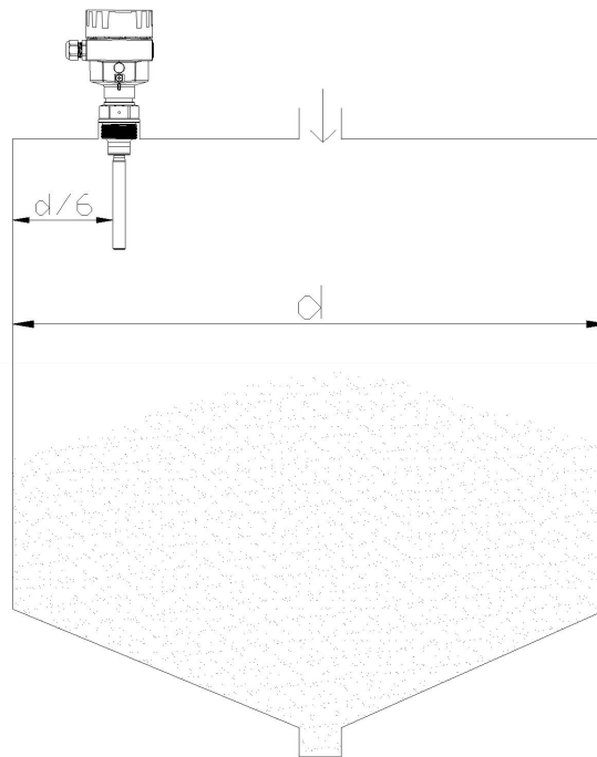
图 4 垂直安装示意图
