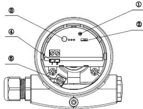
图 10 二线制输出方式
