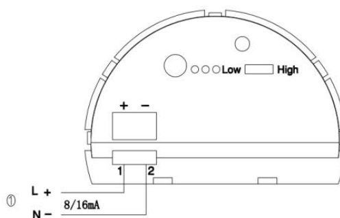
图 8 二线制输出方式
