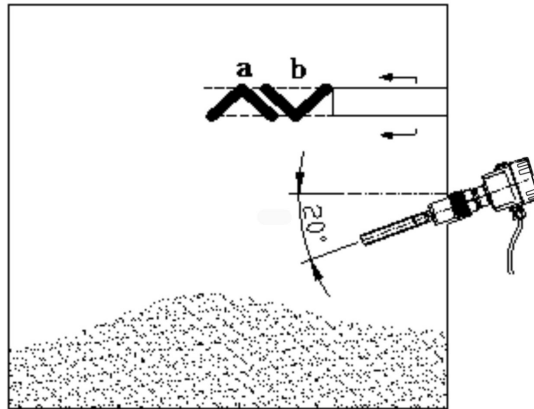
图 2 挡板式安装示意图
